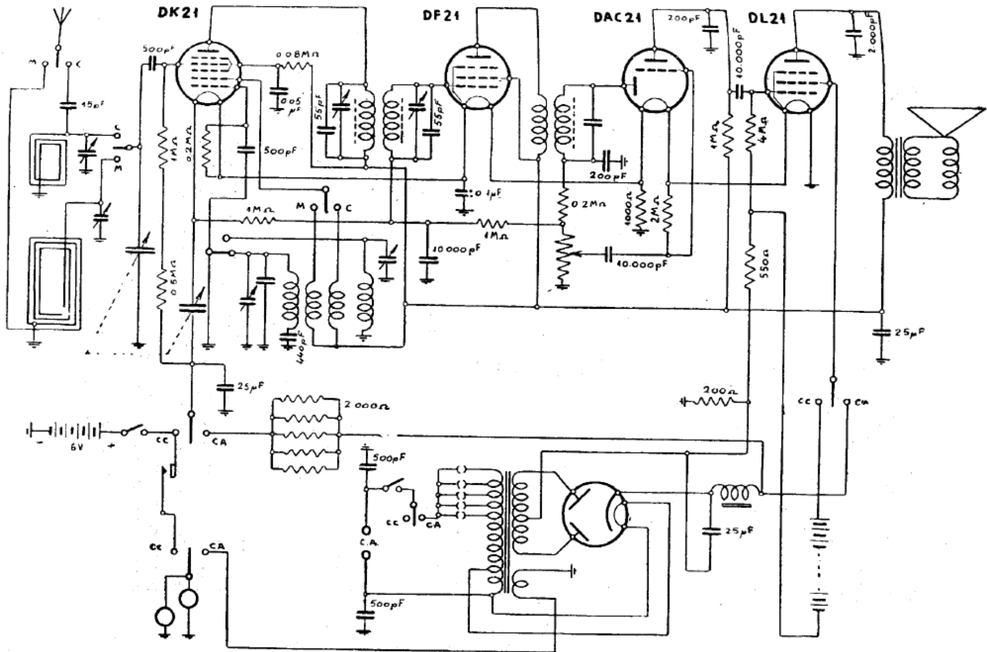
- Phonola mod. 545. Schema complessivo.
